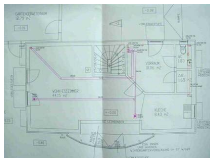
Abbildung 3.145: Einfacher Verlegeplan für die Lüftungsrohre
