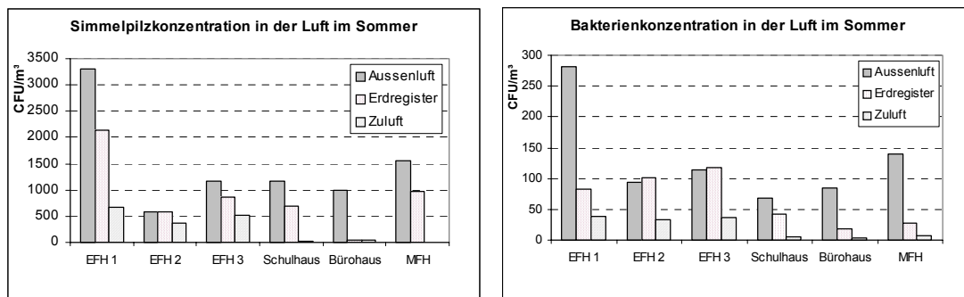
Abbildung 2.51: Schimmelpilz- und Bakterienkonzentration in der Außenluft, im EWT und in der Zuluft der im Sommer untersuchten Anlagen in CFU/m 3 . (CFU=Colony forming unit oder keimbildende Einheit), (Flückiger, 1997)
