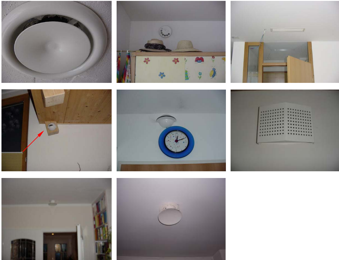
Abbildung 3.132 a- h: Beispiel für Zuluftventile (Induktionslüftung)
