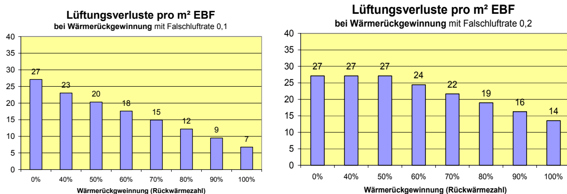
Abbildung 2.39: Rechnerischer jährlicher Heizwärmebedarf pro \text{m}^2 für die Lüftung (Falschluftrate 0,1)
