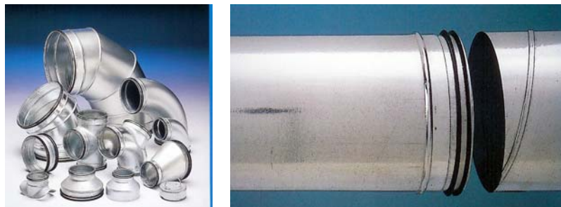
Abbildung 3.143 a-b: Rohrsystem mit Dichtungssystem (Quelle: Fa. Pichler)
